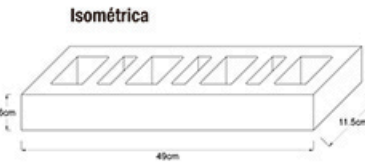
DIMENSIONES EN CM.
