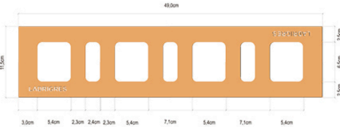
DIMENSIONES EN CM.
